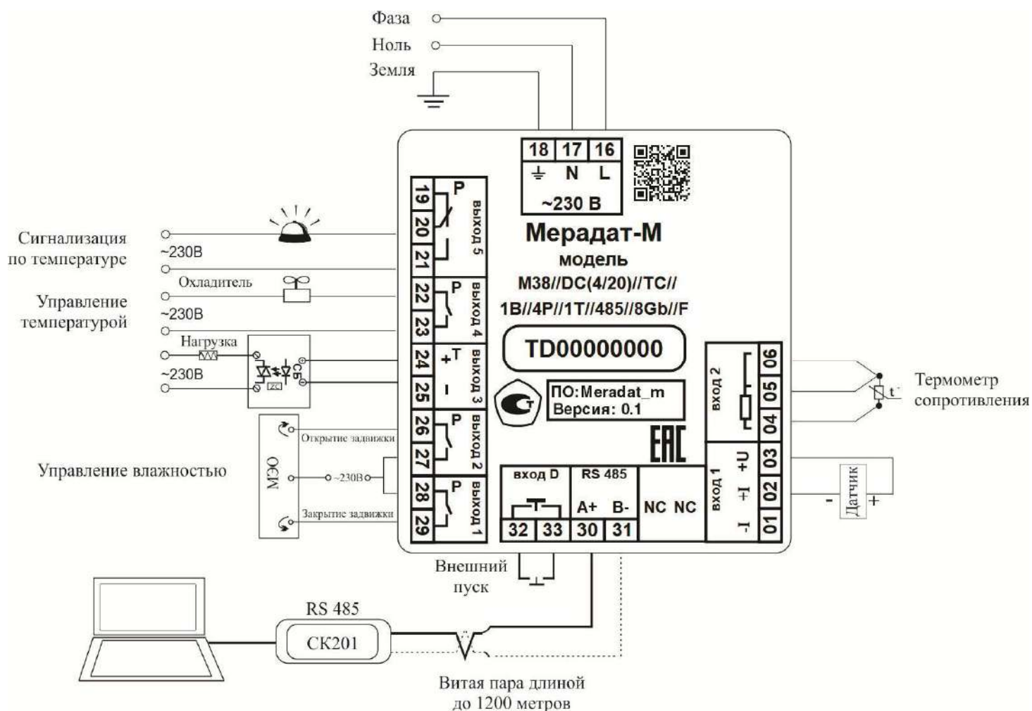
Схема 1. Регулирование влажности с использованием электрозадвижки. регулирование температуры при помощи нагревателя ( N > 1.5 кВт).
